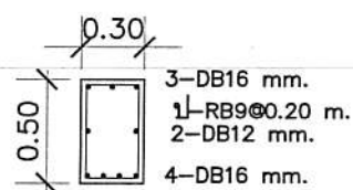
คาน B1 SCALE 1:40
