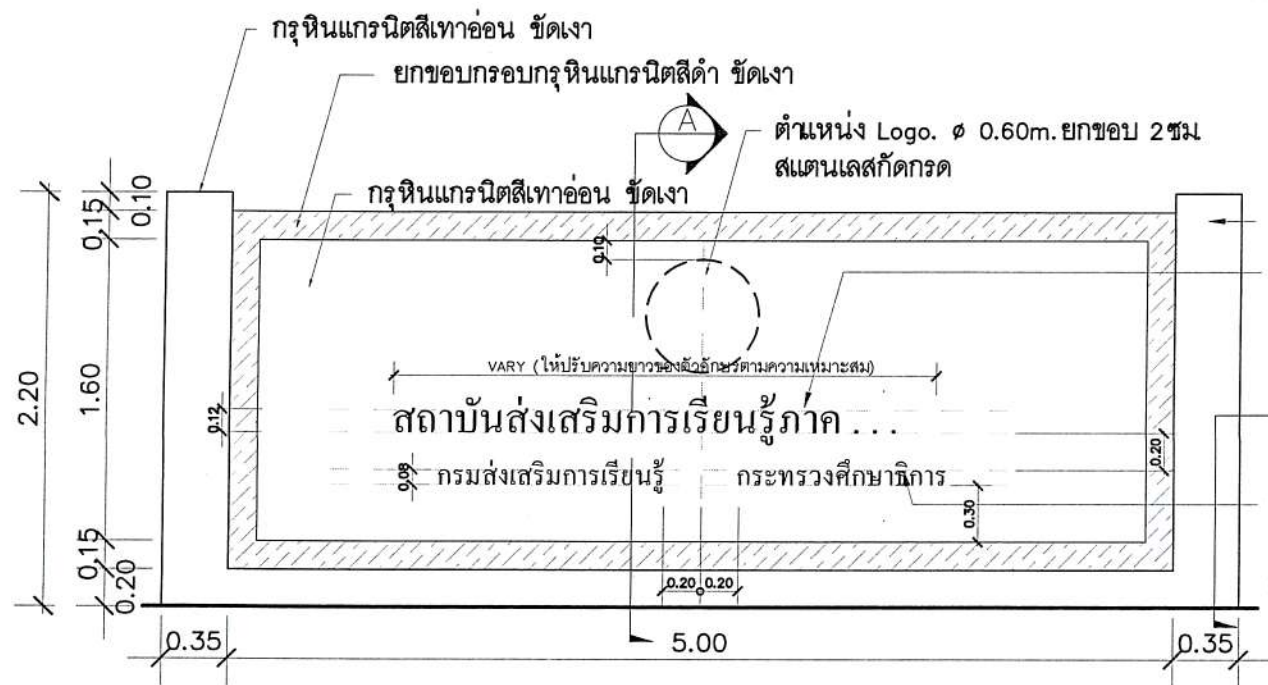
รูปด้านหน้าป้ายชื่อสำนักงาน 5 SCALE 1:40
