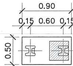
ฐานราก F1 SCALE 1:40
