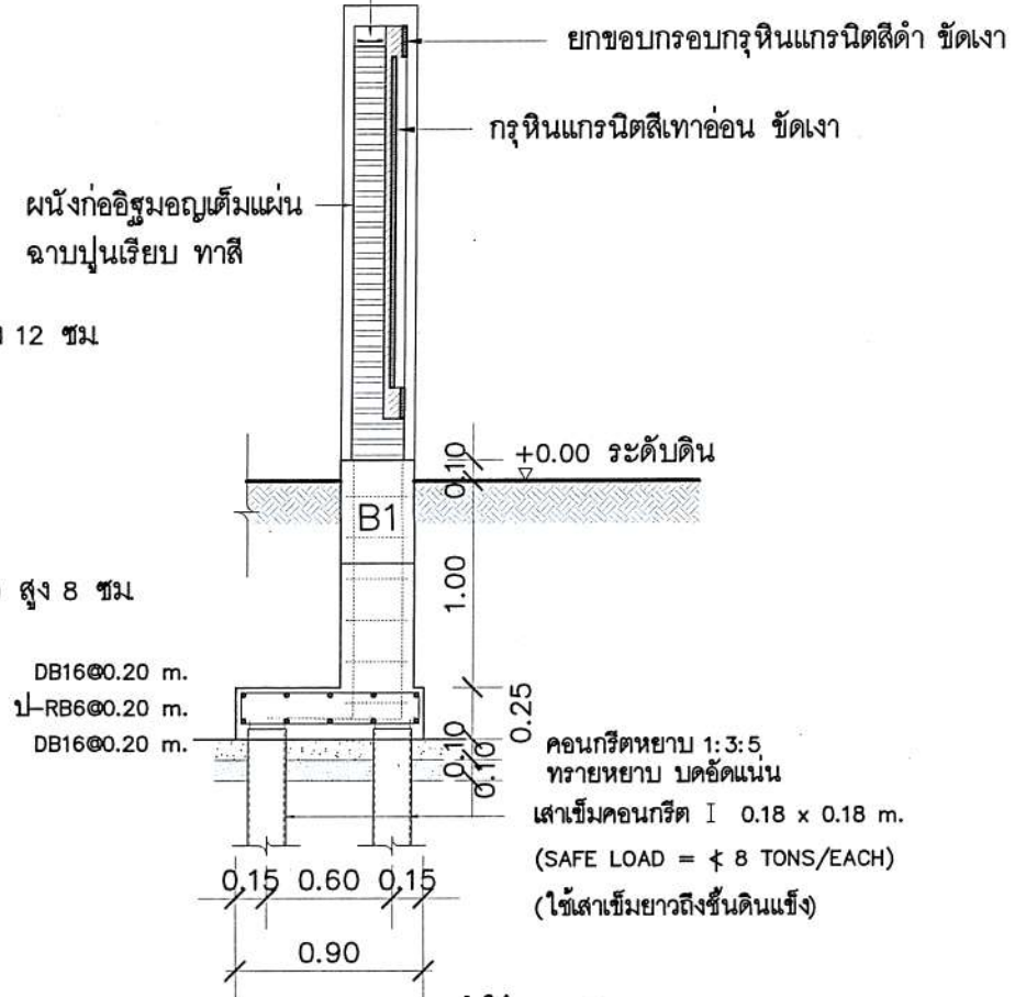
รูปตัด A SCALE 1:40
