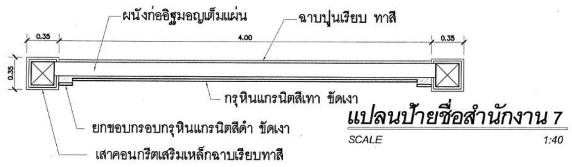
รูปด้านหน้าป้ายชื่อสำนักงาน 7 SCALE 1:40
