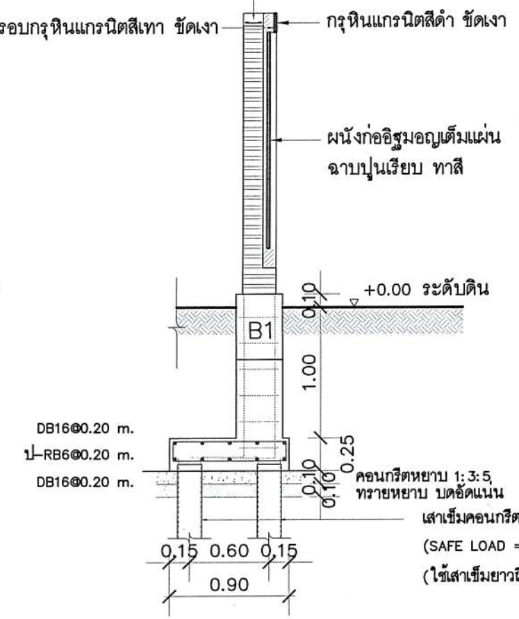
รูปตัด A SCALE 1:40
