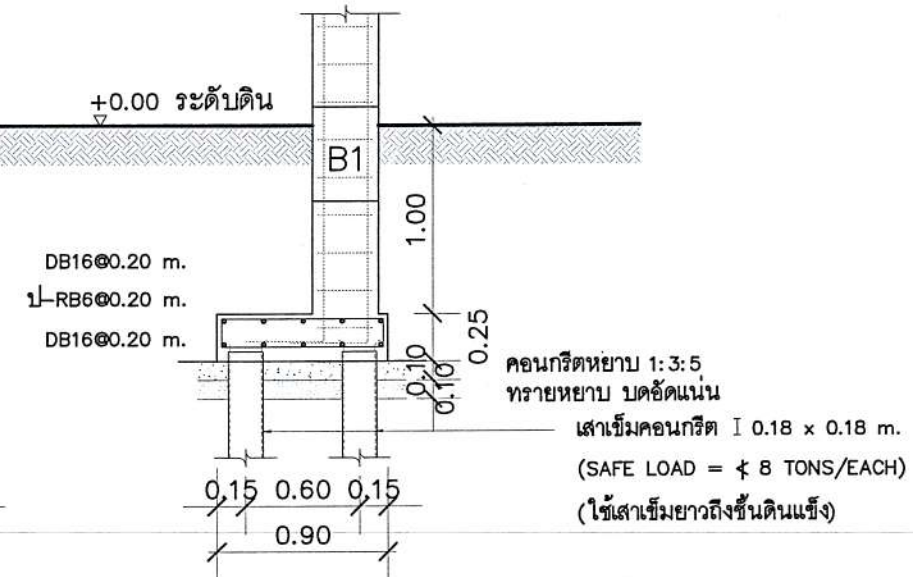
รูปตัด A SCALE 1:40
