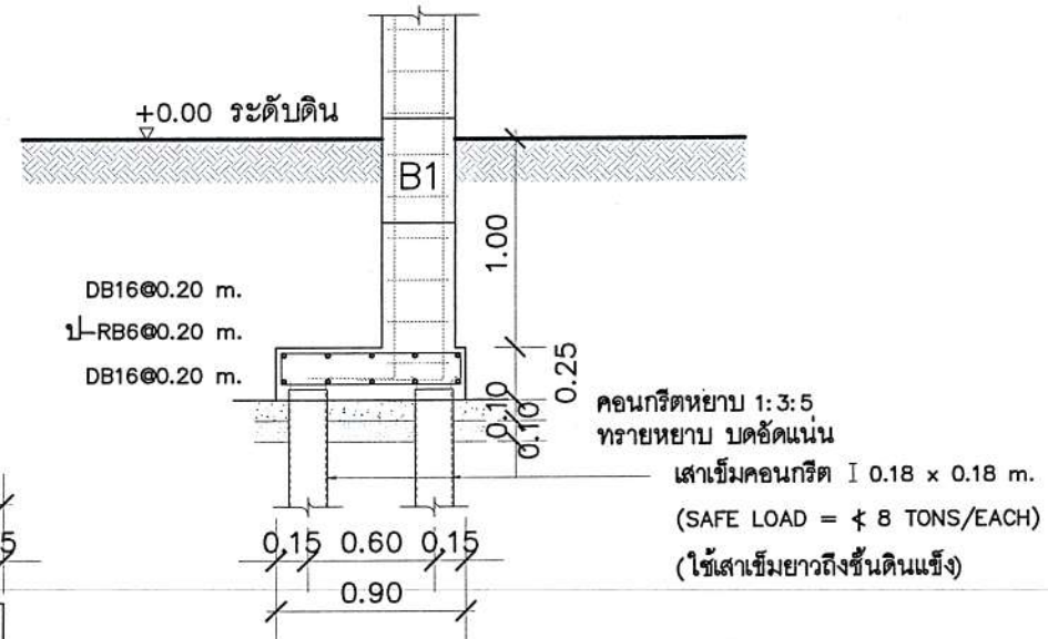
รูปตัด A SCALE 1:40
