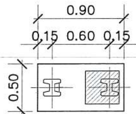
ฐานราก F1 SCALE 1:40
